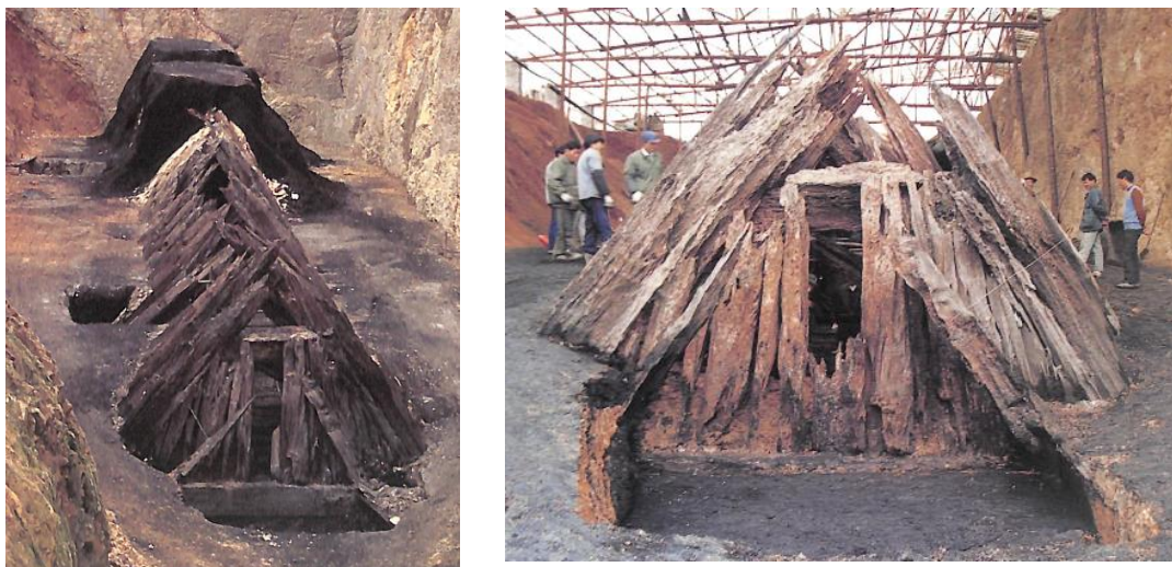
圖 7 印山越王陵墓室 《印山越王陵》，彩版 15、19。
