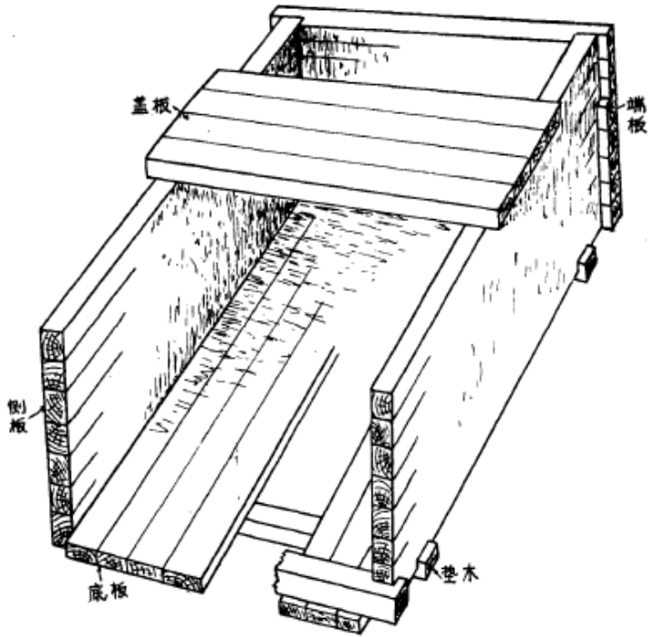
圖 4 晉侯墓 M1 外槨復原圖 〈1992 年春天馬 - 曲村遺址墓葬發掘報告〉，頁 15。
